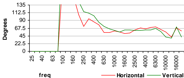
Beamwidth
