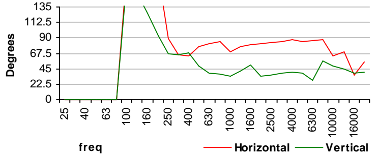
Beamwidth
