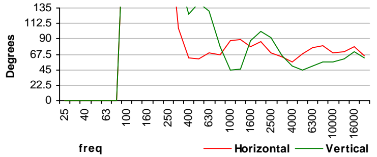
Beamwidth
